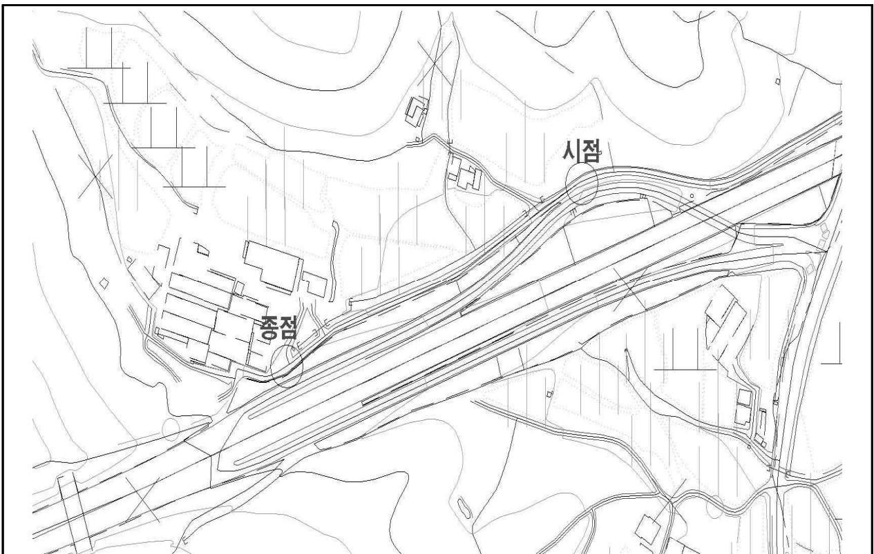
&lt;그림 2.3.1&gt; 설계도면 선형과 금회 실측 값 비교
